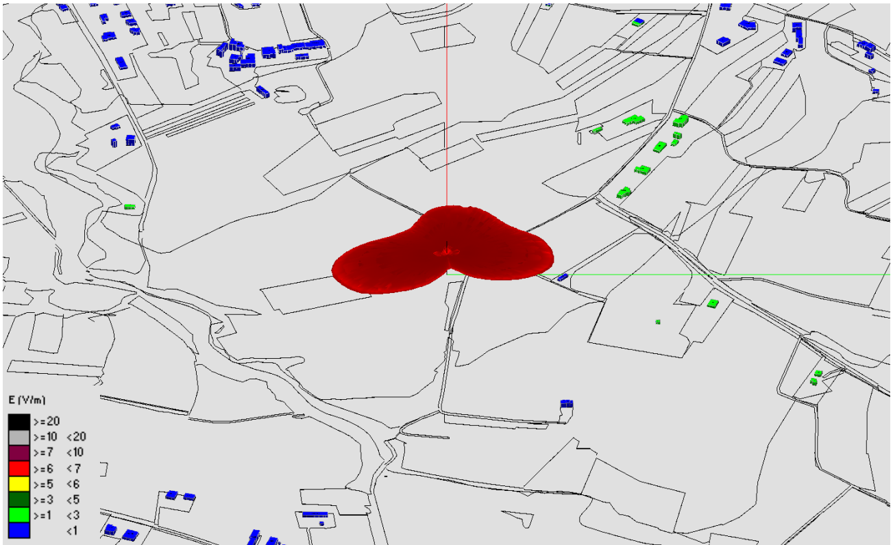
Fig. 2 Impatto Elettromagnetico – zona Via del Colletto – 0° N
