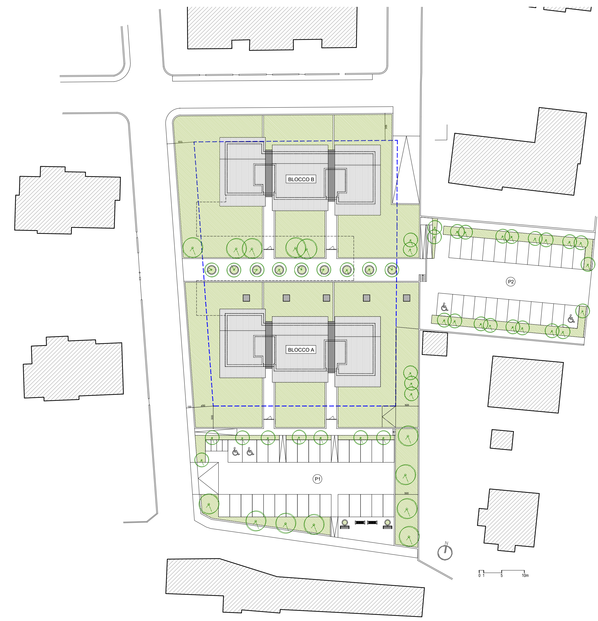
PLANIMETRIA PROGETTO
