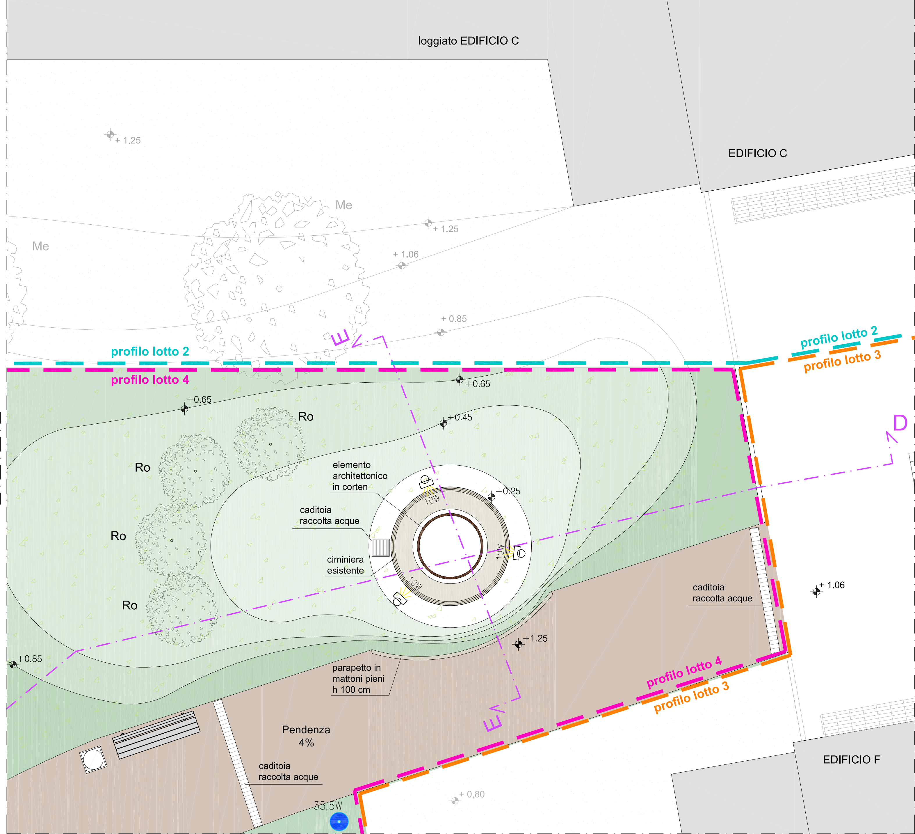
STRALCIO PLANIMETRIA - scala 1:50
