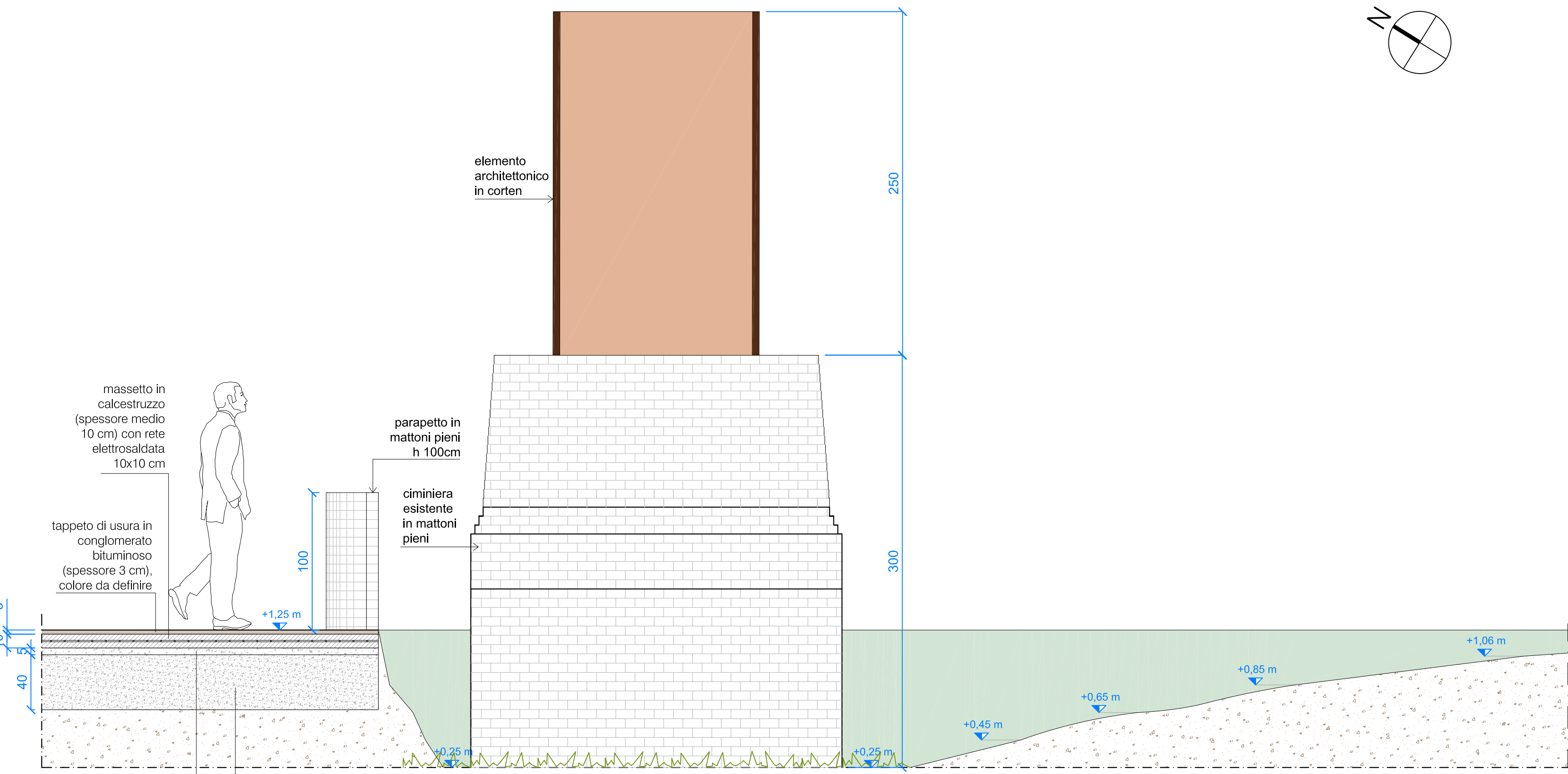
PROSPETTO - scala 1:25
