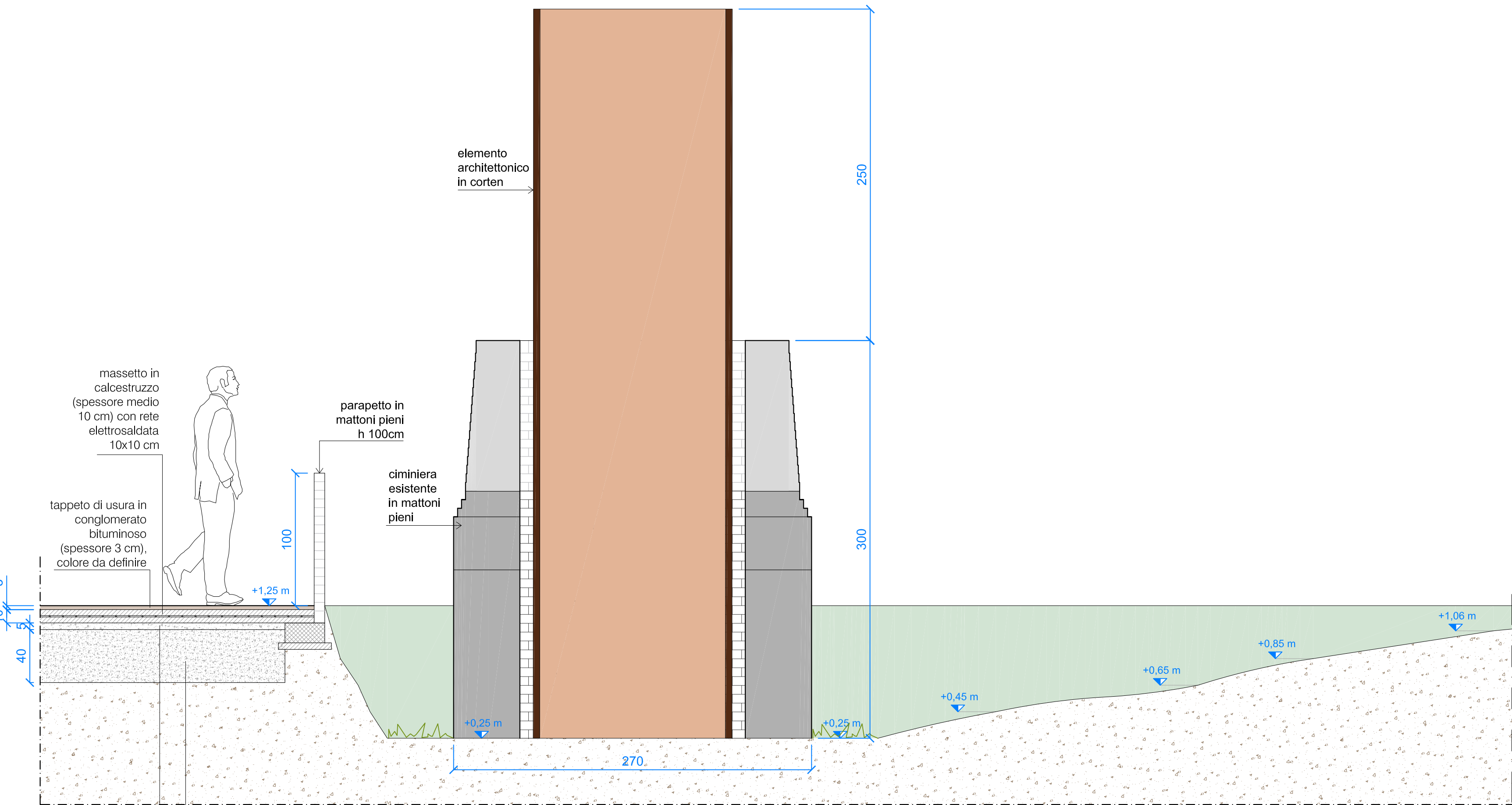
PARTICOLARE SEZIONE E-E - scala 1:25
