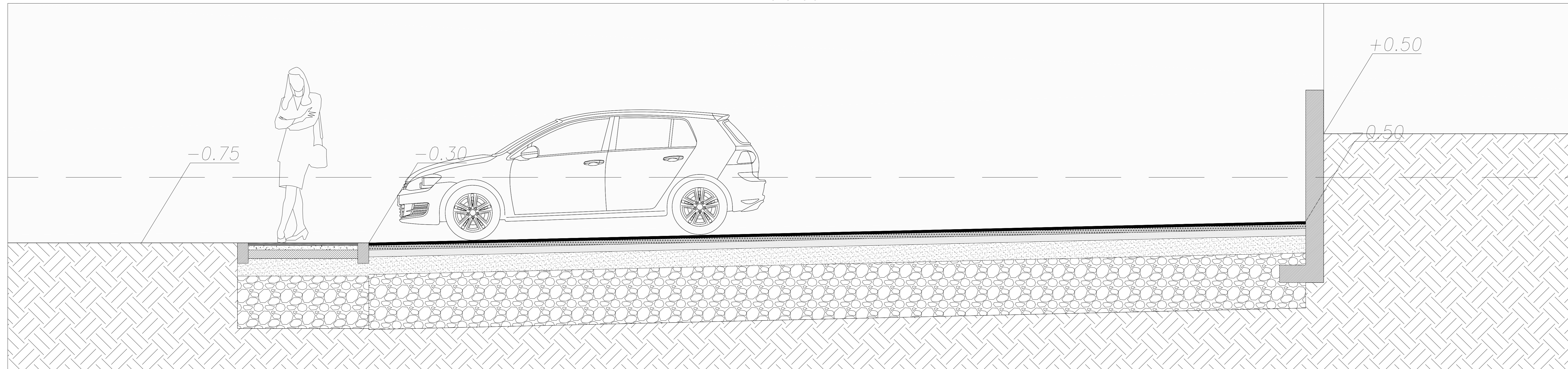
SEZIONE C - C
