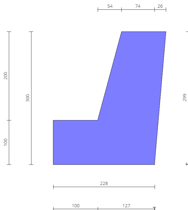
Figura 9 – Estratto dal software di calcolo MAX 16.0 – Sezione di verifica
