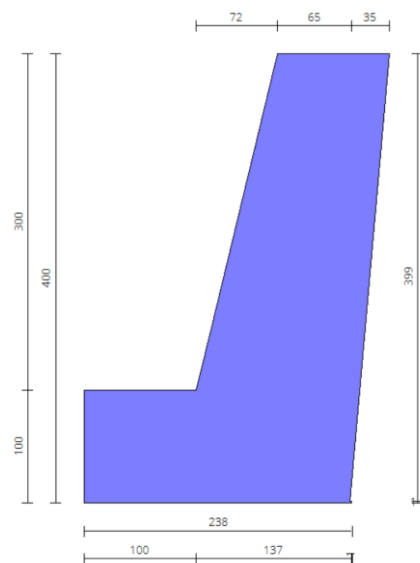
Figura 15 - Estratto dal software di calcolo MAX 16.0 - Sezione di verifica
