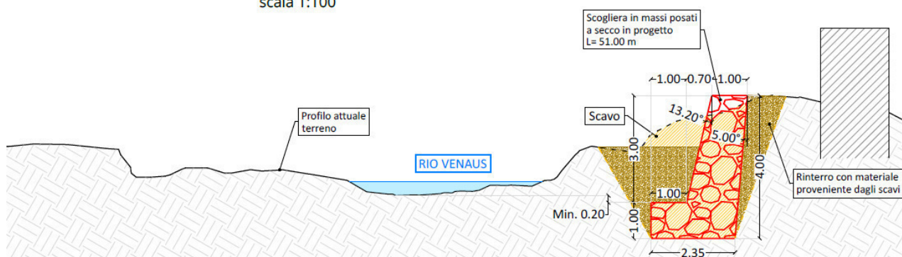
Figura 14: Sezione generica per il modello di calcolo.
