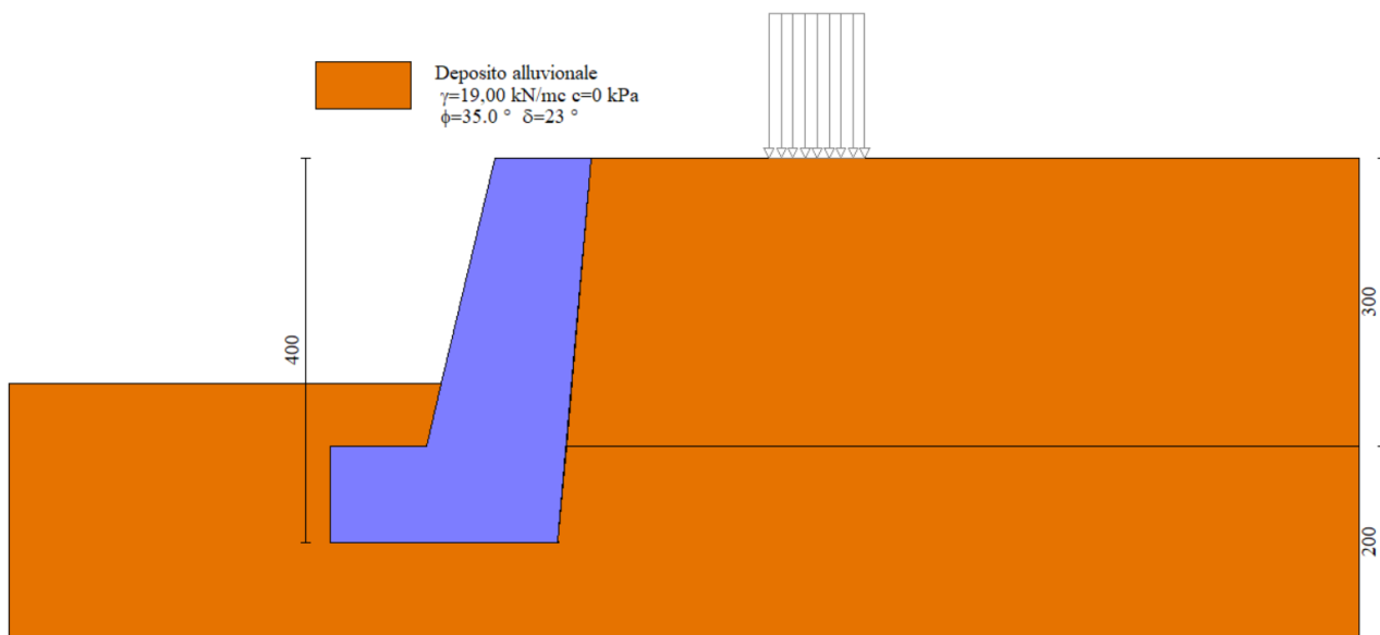
Figura 16 - Estratto dal software di calcolo MAX 16.0 - Sezione di verifica
