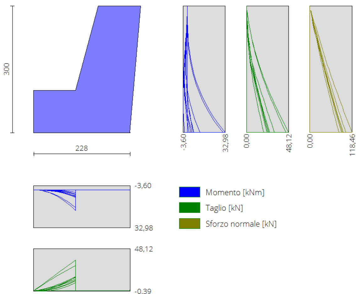
Figura 11: Involuppo sollecitazioni agenti–Momento [kNm], Taglio [kN], Sforzo normale [kN].
