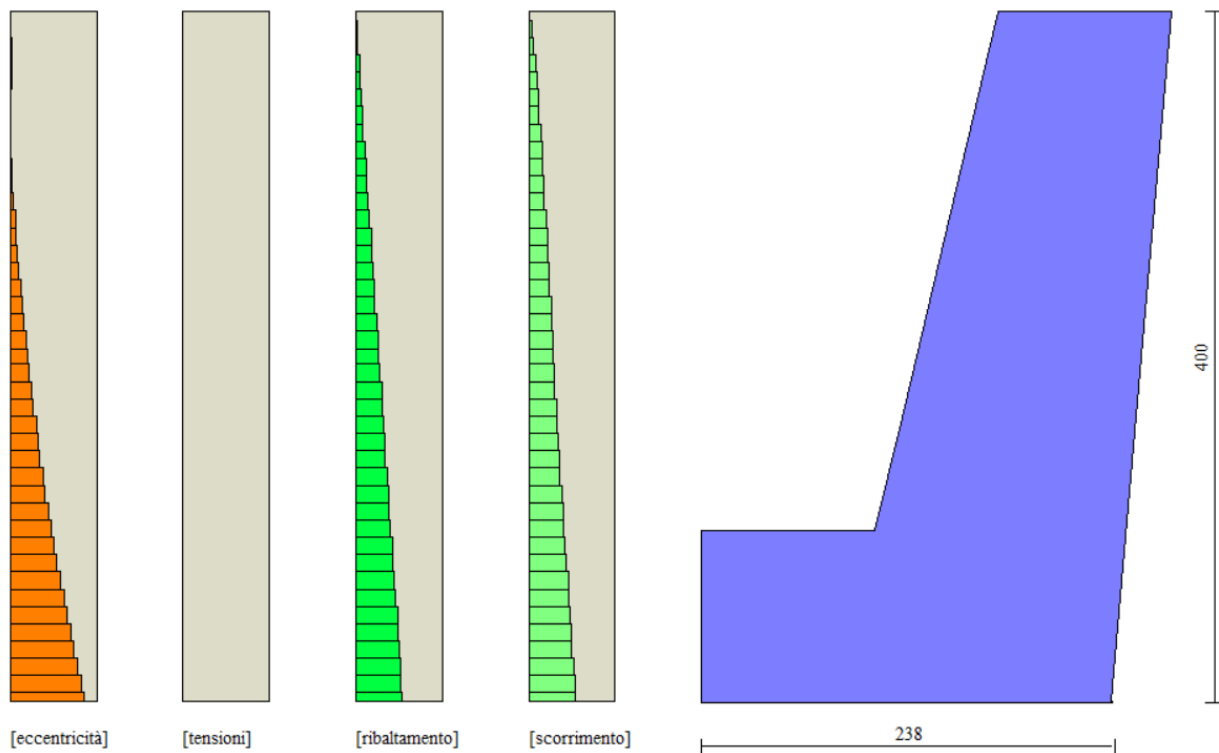
Figura 19. Verifiche muro a gravità.
