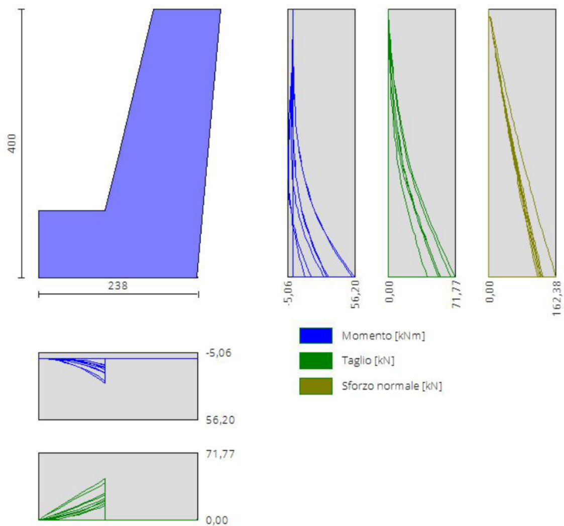
Figura 17: Involuppo sollecitazioni agenti–Momento [kNm], Taglio [kN], Sforzo normale [kN].
