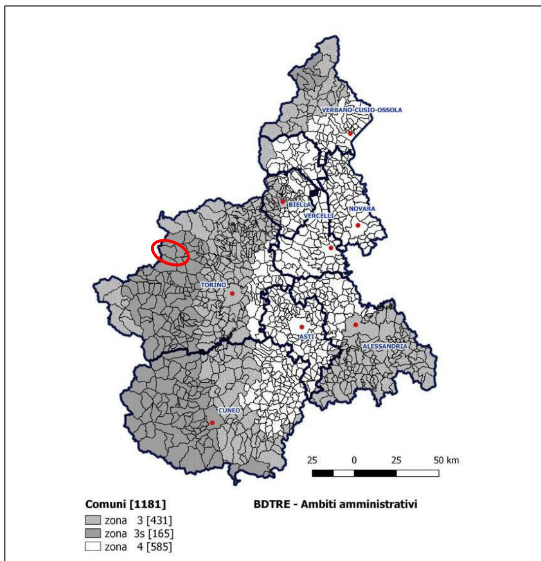
Figura 7 - Mappatura delle aree sismiche in Piemonte.
