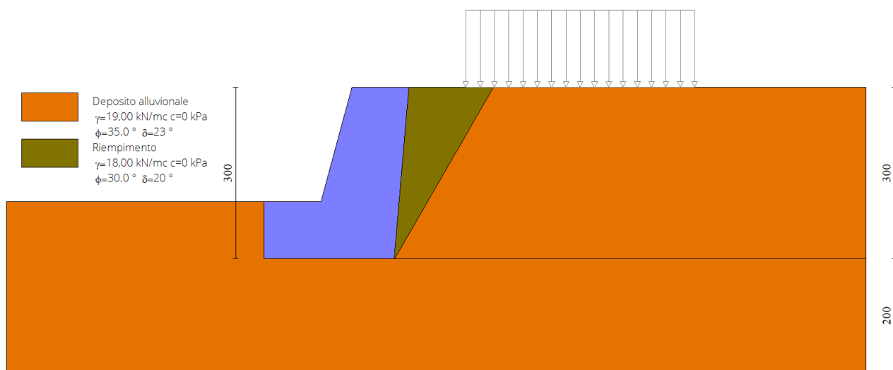
Figura 10 - Estratto dal software di calcolo MAX 16.0 – Sezione di verifica
