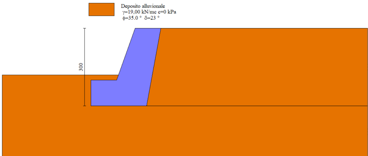
Figura 22 - Estratto dal software di calcolo MAX 16.0 - Sezione di verifica
