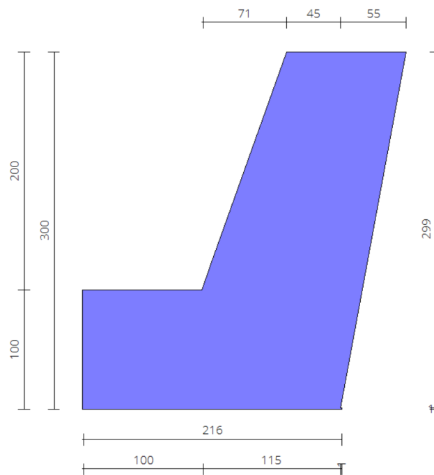
Figura 21 - Estratto dal software di calcolo MAX 16.0 - Sezione di verifica
