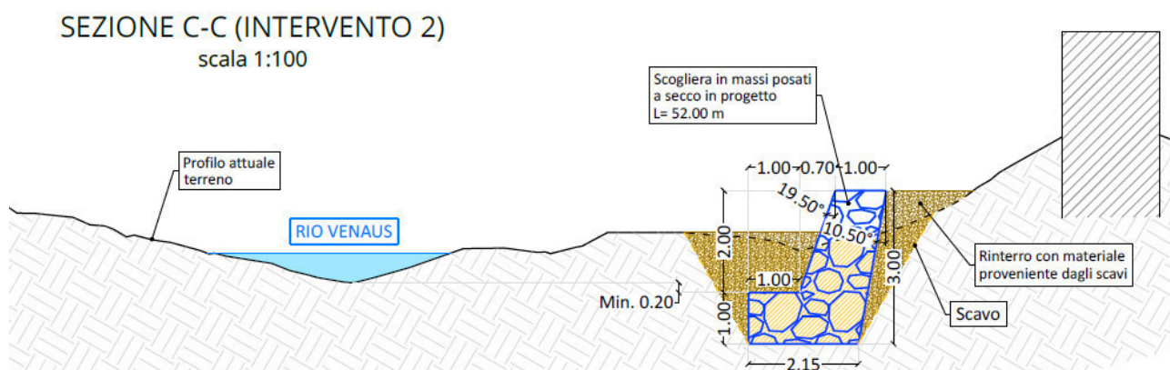
Figura 20: Sezione generica per il modello di calcolo.
