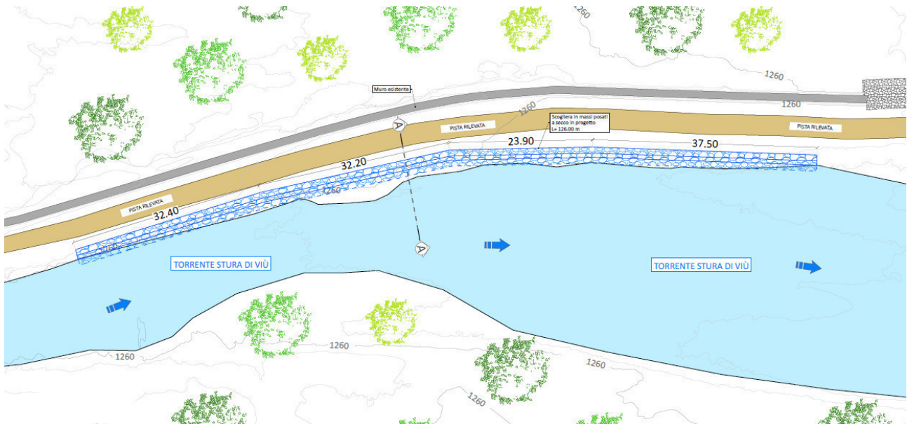
Figura 3 – Estratto della tavola 05.1 - Planimetria di progetto Intervento 1
