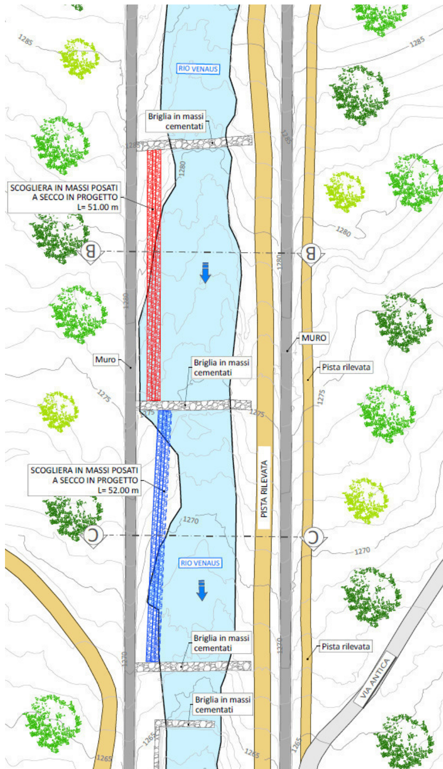
Figura 5 - Estratto della tavola 05.2 - Planimetria di progetto Intervento 2
