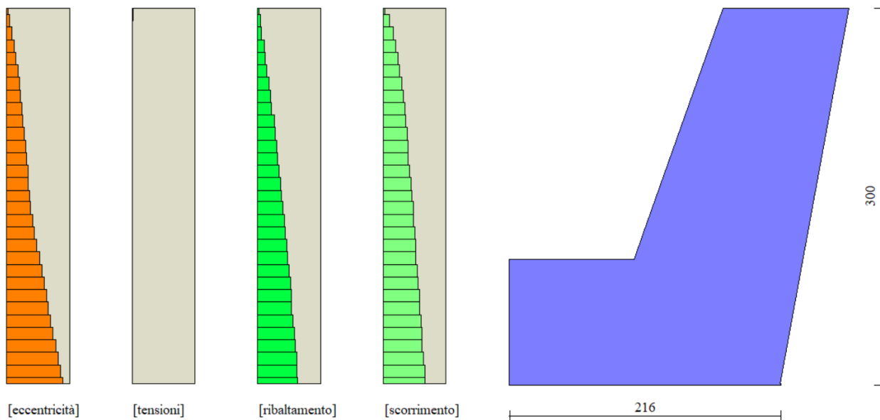
Figura 25. Verifiche muro a gravità.
