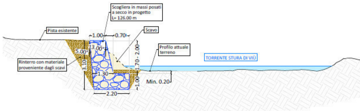
Figura 4 – Estratto della tavola 06 - Sezioni di progetto
