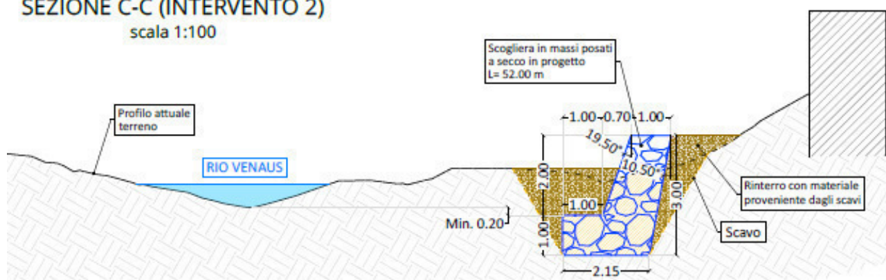
Figura 6 – Estratto della tavola 06 - Sezioni di progetto
