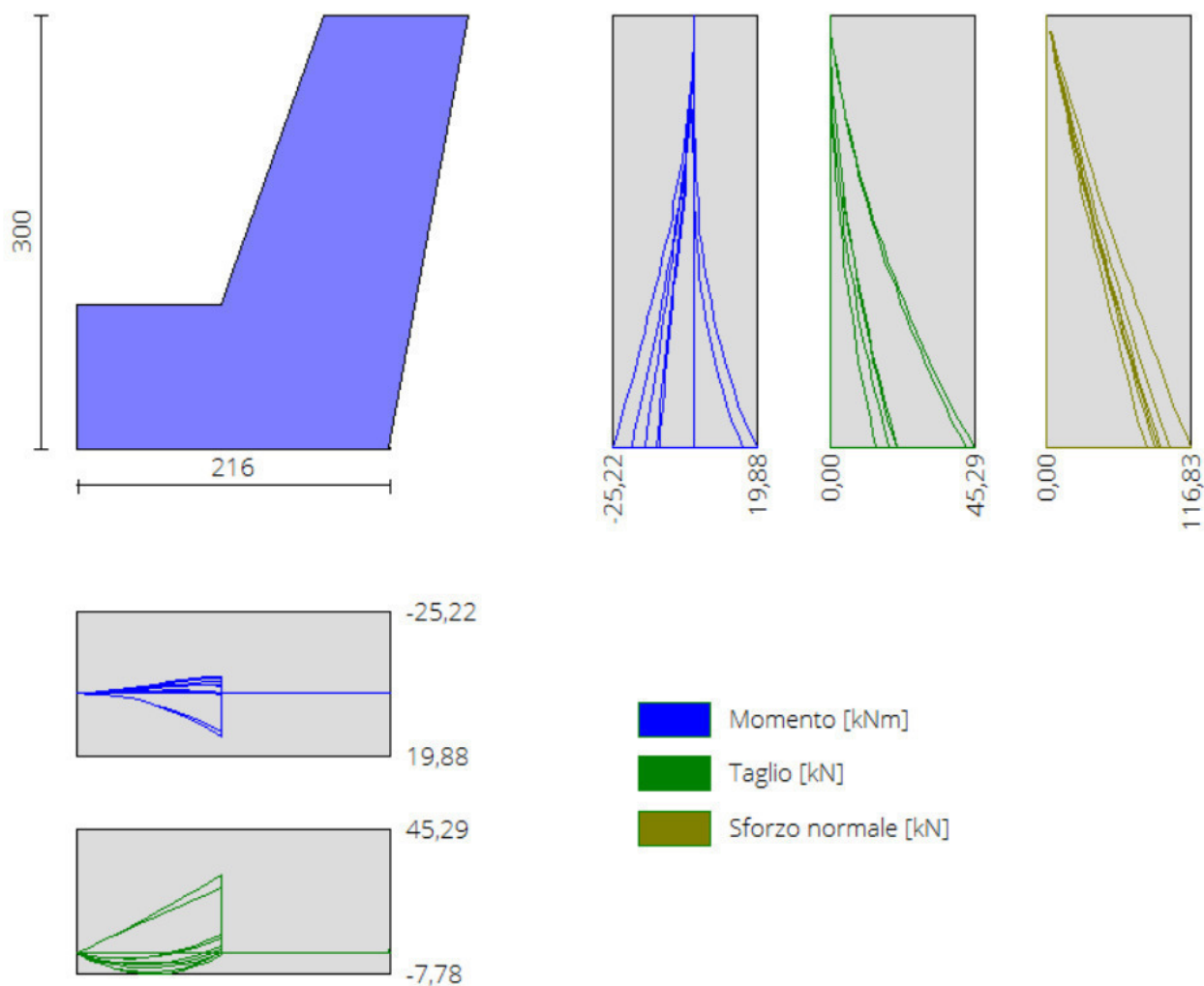
Figura 23: Involuppo sollecitazioni agenti–Momento [kNm], Taglio [kN], Sforzo normale [kN].
