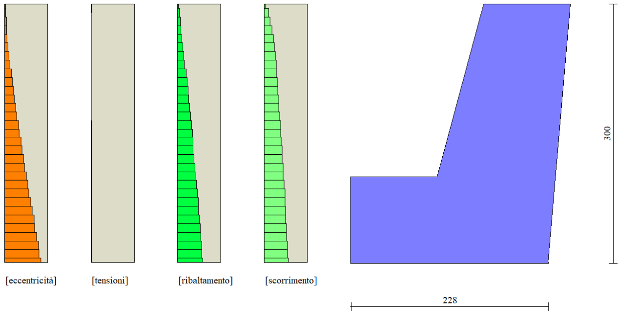
Figura 13. Verifiche muro a gravità.
