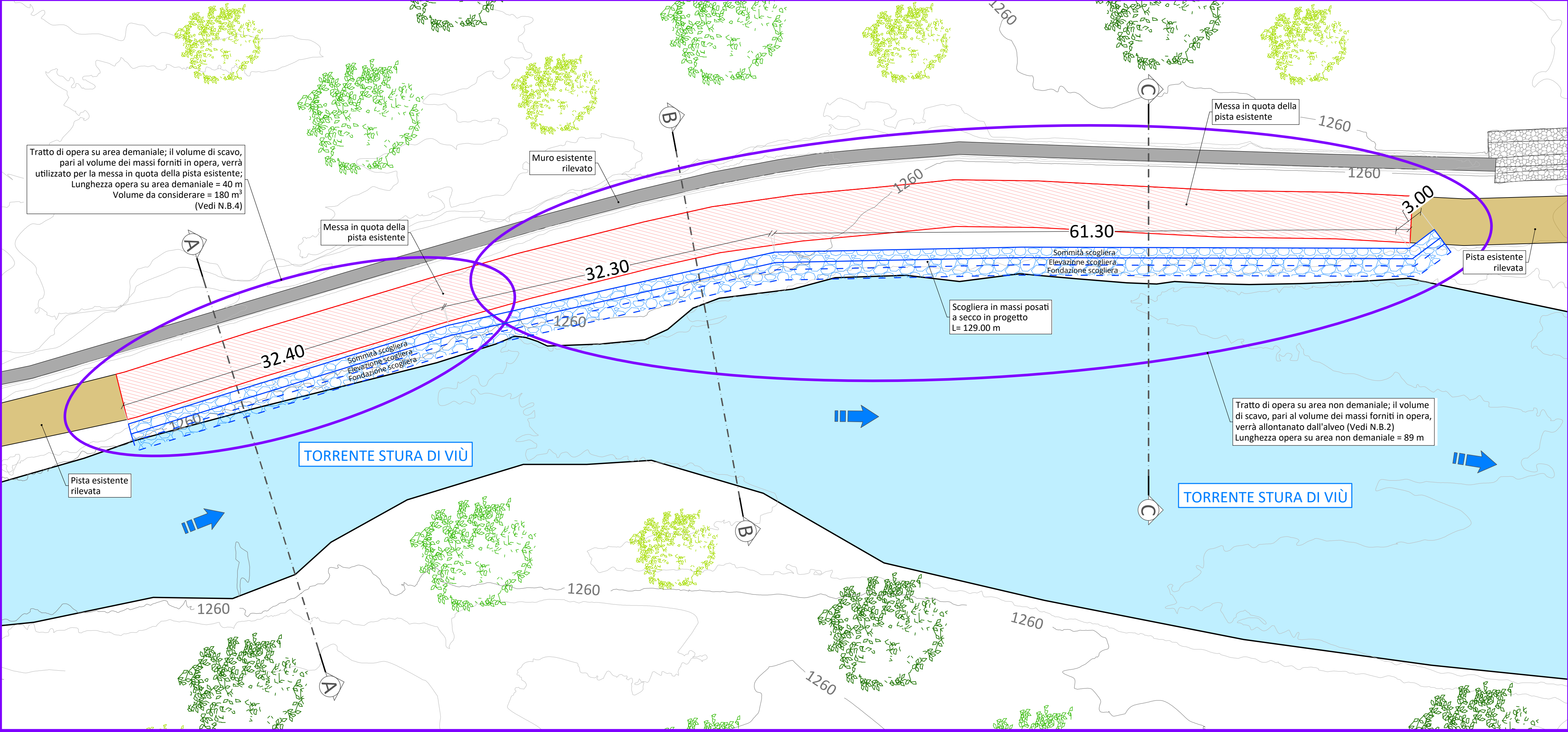
INGRANDIMENTO PLANIMETRIA DI PROGETTO - INTERVENTO 1 scala 1:250
