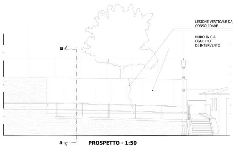
PROSPETTO - 1:50
