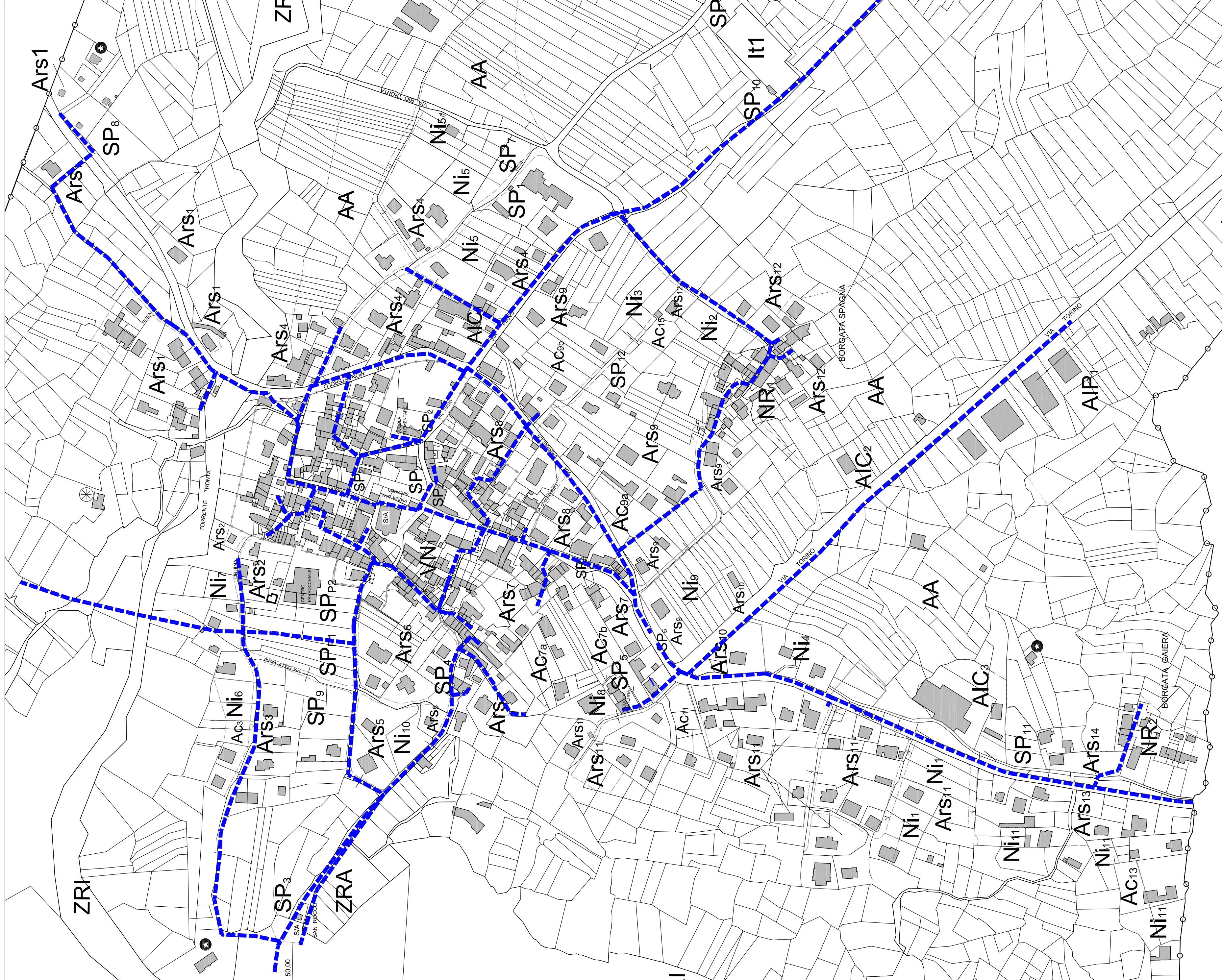
RETE ACQUEDOTTO Concentrico e nuclei rurali
