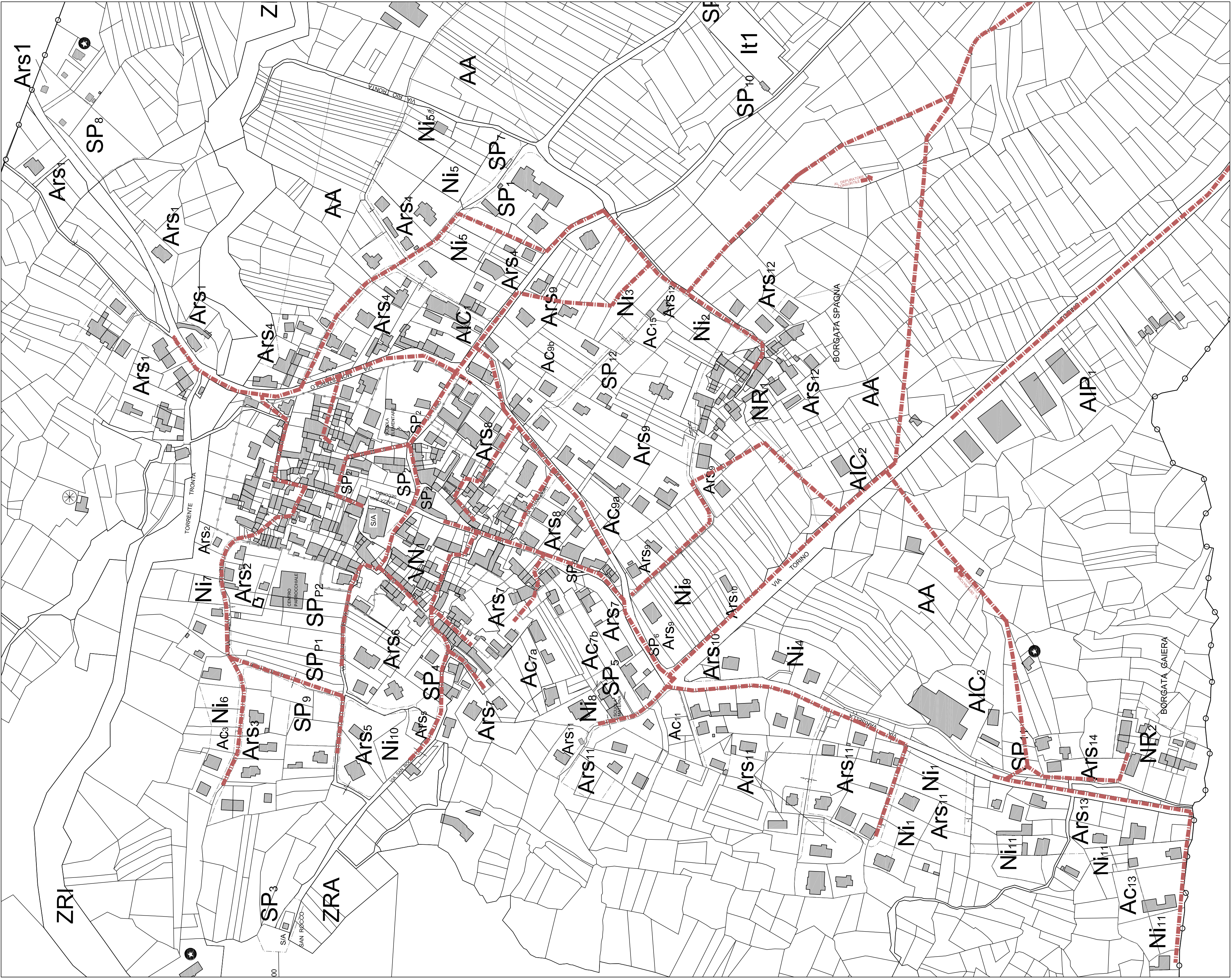
RETE FOGNARIA 1 (NERA O MISTA) Concentrico e nuclei rurali
