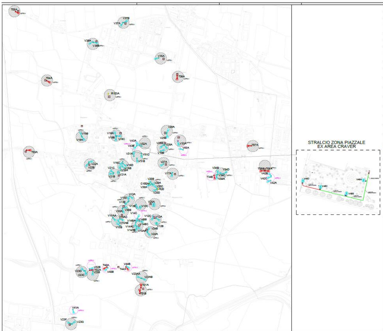
Planimetria generale varchi.
