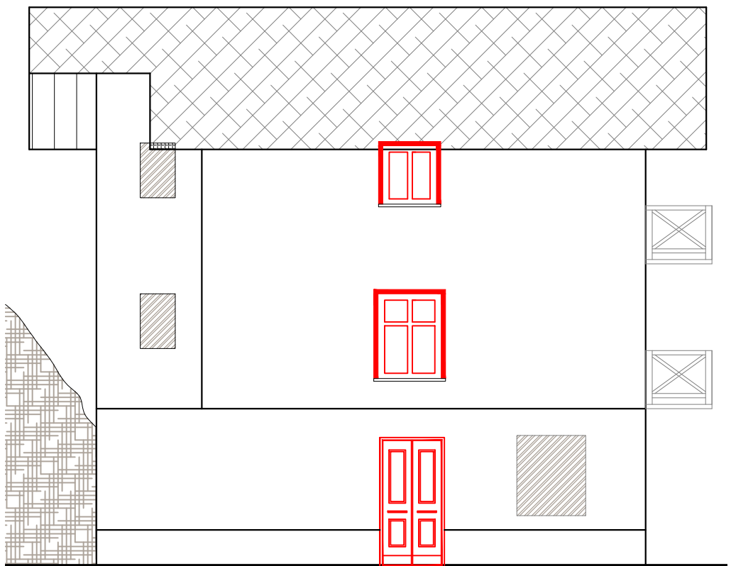
PROSPETTO OVEST
