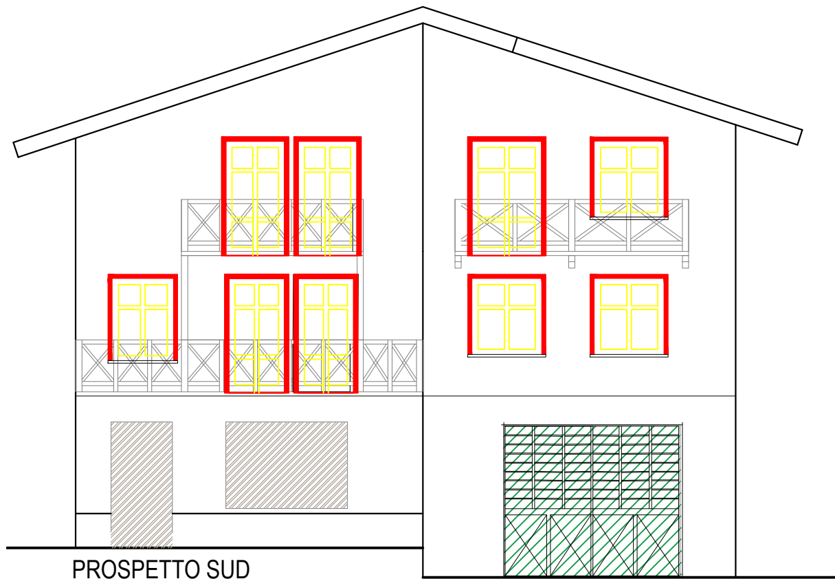
PROSPETTO SUD
