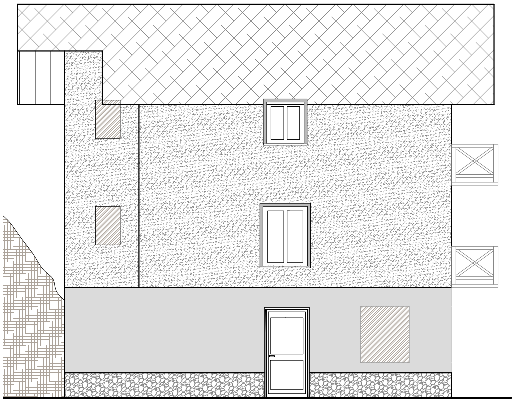
PROSPETTO OVEST
