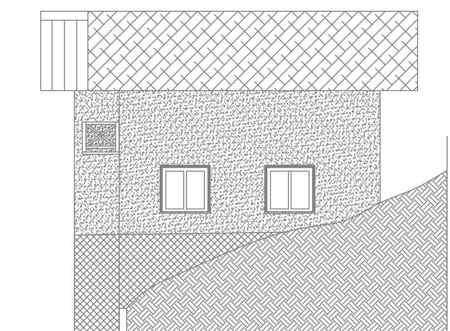
PROSPETTO EST scala 1:100
