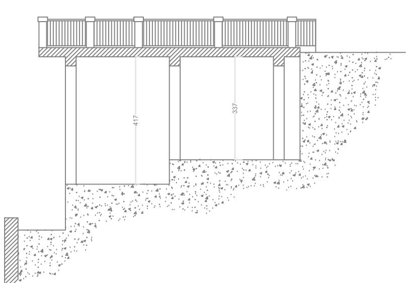
SEZIONE 1-1 scala 1:100
