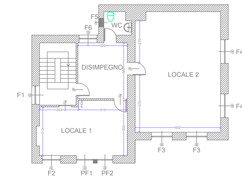
PLANIMETRIA PIANO PRIMO scala 1:100
