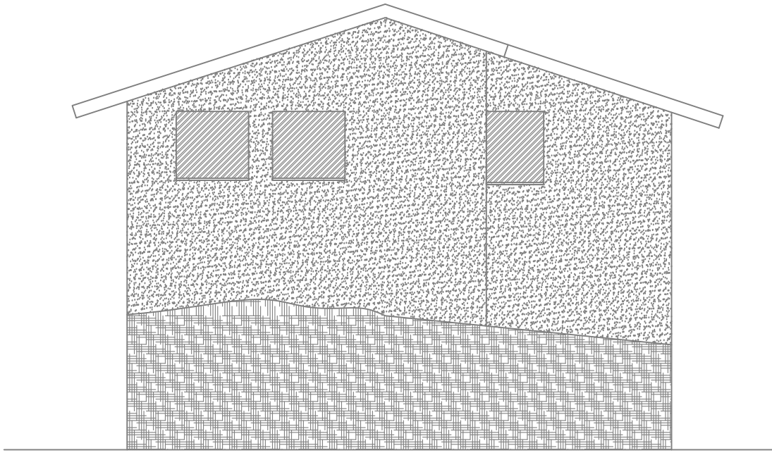
PROSPETTO NORD scala 1:100
