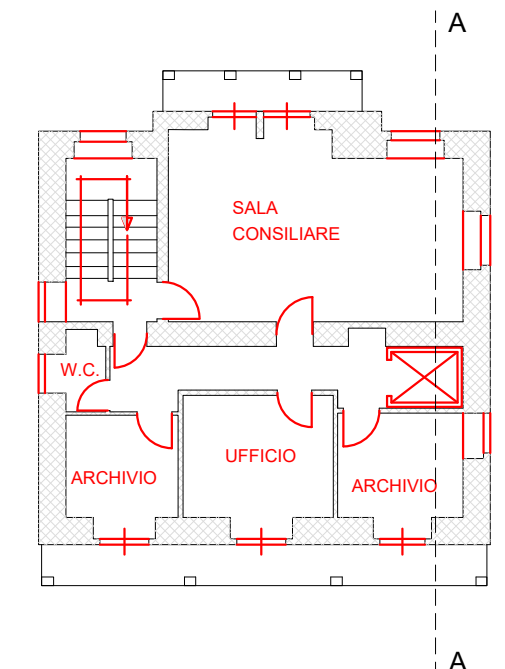
PLANIMETRIA PIANO PRIMO scala 1:100
