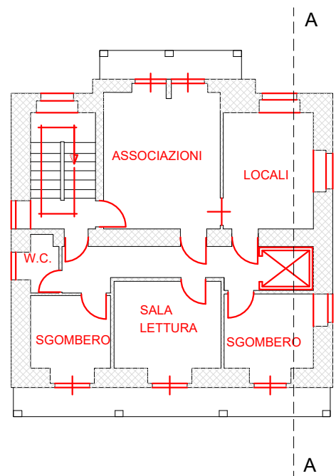
PLANIMETRIA PIANO SECONDO scala 1:100
