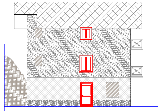
PROSPETTO OVEST scala 1:100
