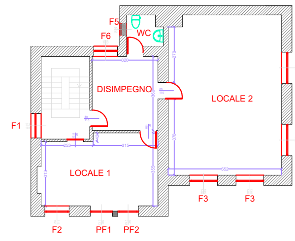
PLANIMETRIA PIANO PRIMO scala 1:100
