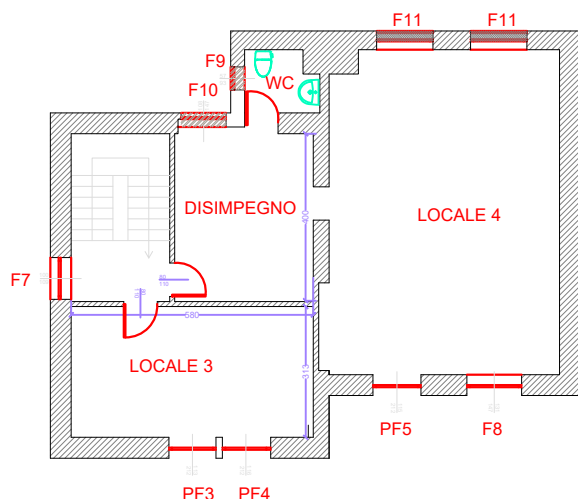
PLANIMETRIA PIANO SECONDO scala 1:100
