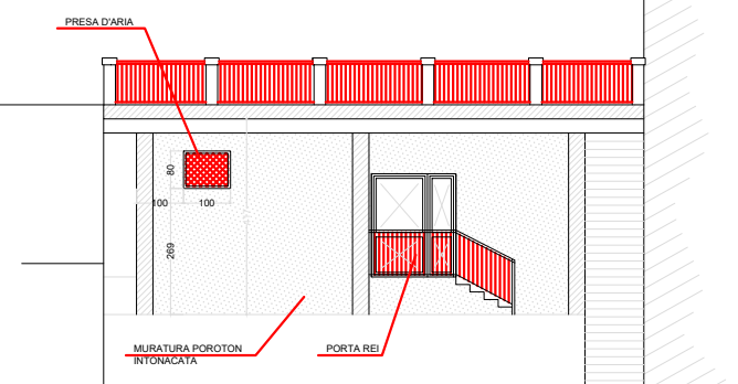
PROSPETTO scala 1:100
