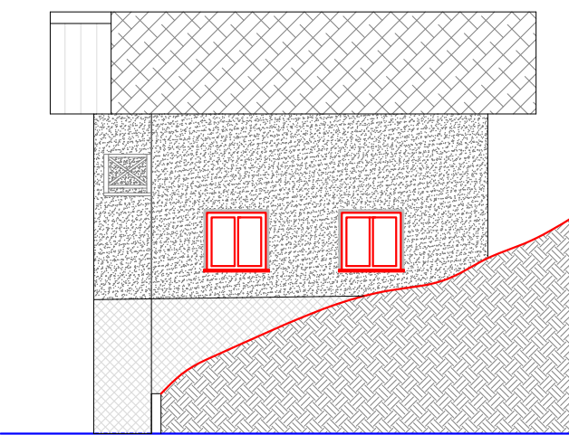
PROSPETTO EST scala 1:100
