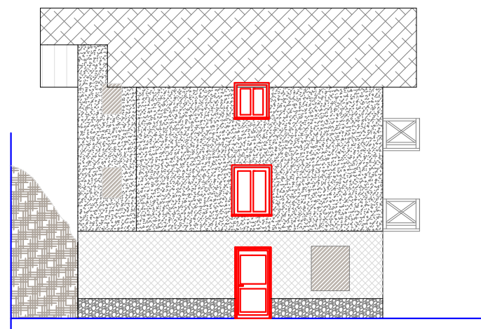
PROSPETTO OVEST scala 1:100
