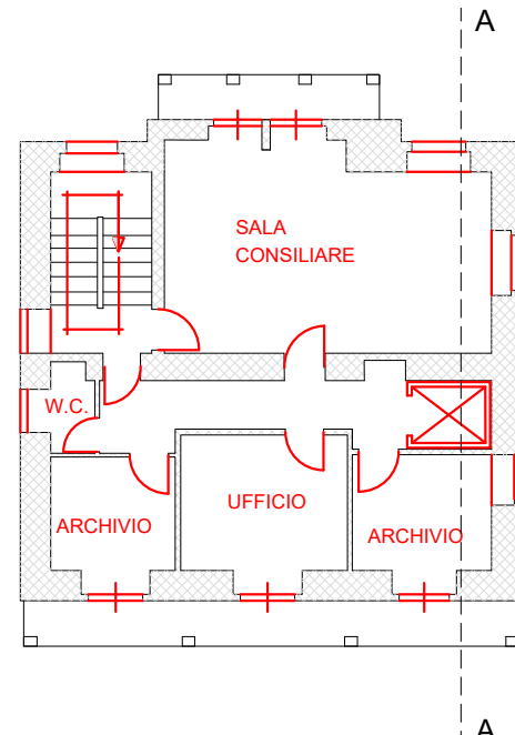
PLANIMETRIA PIANO PRIMO scala 1:100
