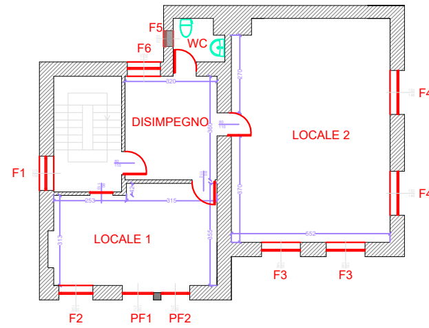
PLANIMETRIA PIANO PRIMO scala 1:100
